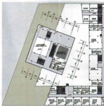
4 三层平面
