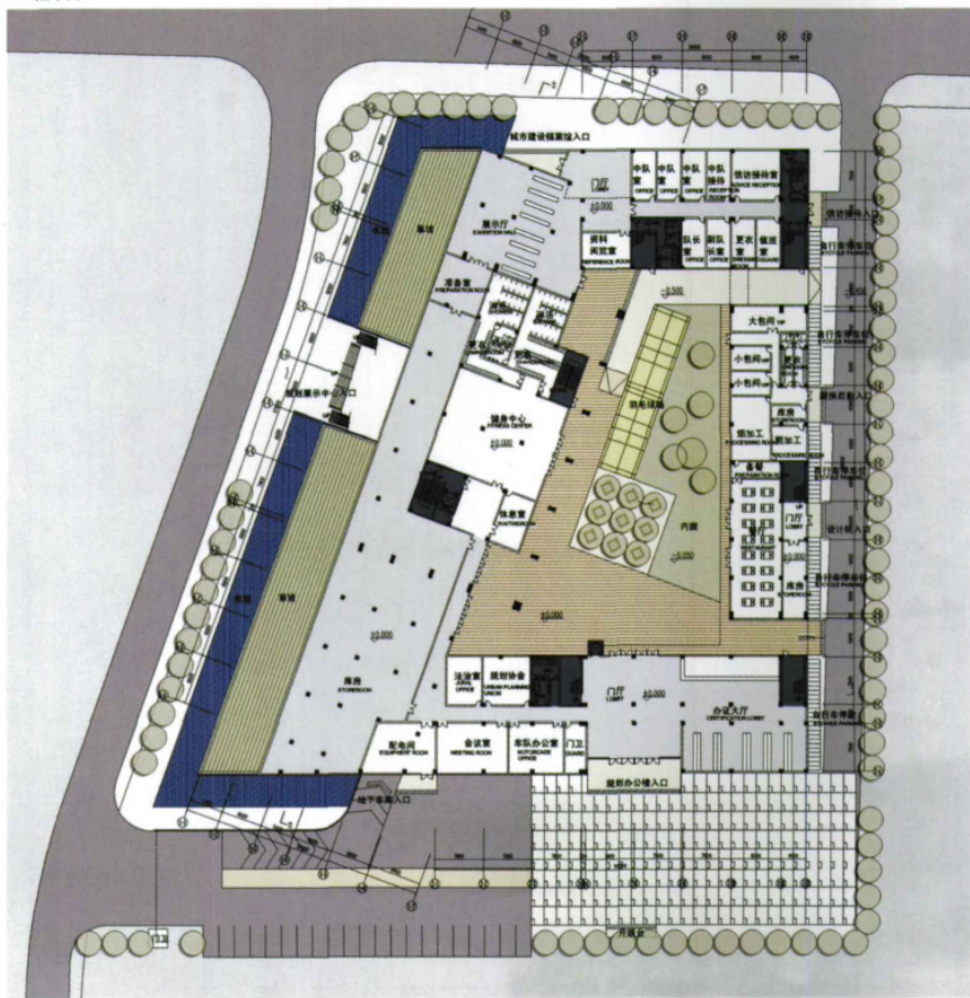
2 一层平面
